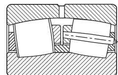
Рис. 8. Сепаратор на распорках.
