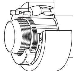
Рис. 26. Гидравлическая гайка при демонтаже стяжной втулки.
