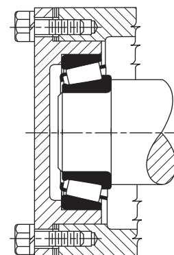
Со стаканом наружного кольца. Площадь поперечного сечения стакана должна быть в среднем равна площади сечения наружного кольца подшипника.
