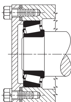
С толкателем наружного кольца.
