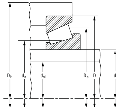
Рис. 15. Размерные параметры, влияющие на регулировку зазора под действием посадки и температуры.
