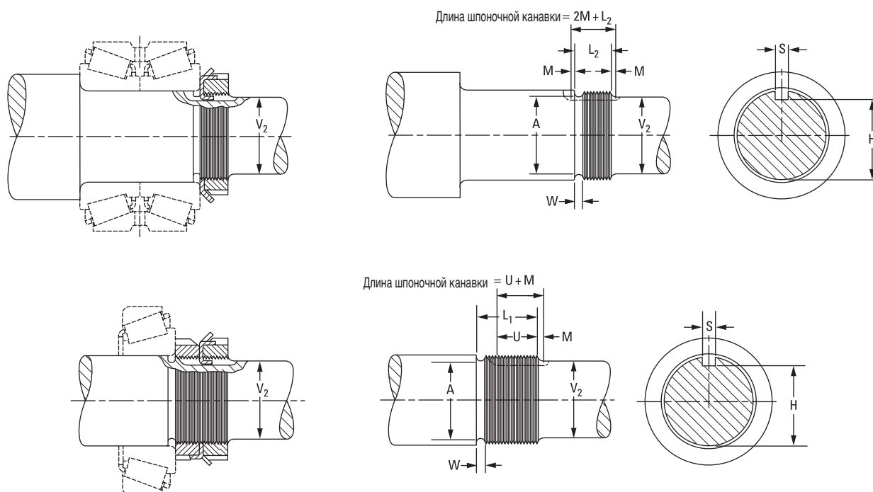
Рис. 56. Стопорные гайки, стопорные шайбы и стопорные шайбы с внутренним выступом.
