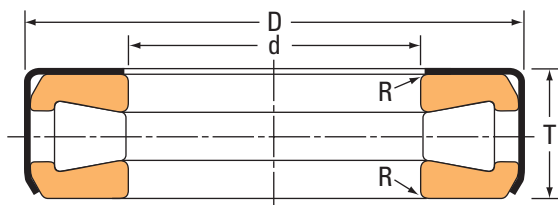
Рис. В. ИСПОЛНЕНИЕ TTCS.
