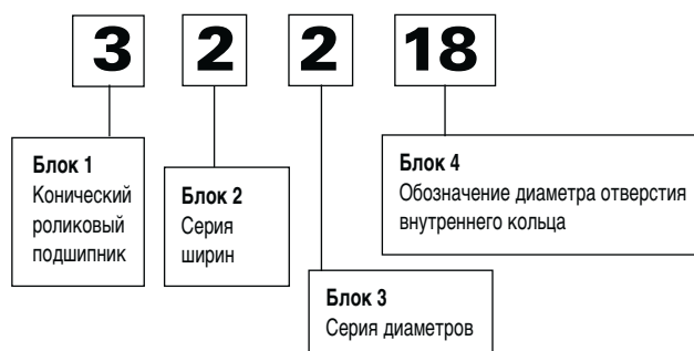
Рис. 30. Оригинальная система обозначений ISO.
